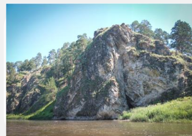
Геологический разрез Аргус
